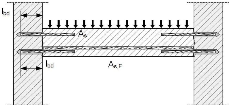
Figure A3: Ancrage d'armatures en extrémité de dalles ou poutres, dimensionné en tenant compte des exigences d'adhérence partielle
