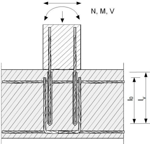
Figure A3: Ancrage d'armatures en extrémité de dalles ou poutres, dimensionné en tenant compte des exigences d'adhérence partielle
